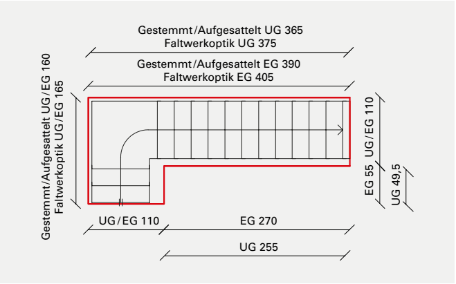
1 x 1/4 gewendelte Treppe, 2-läufige Podesttreppe
