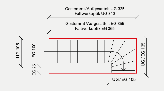
1 x 1/4 gewendelte Treppe
