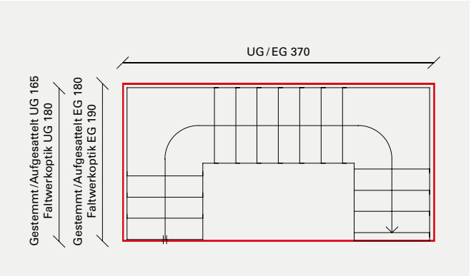
2 x 1/4 gewendelte Treppe, 3-läufige Podesttreppe
