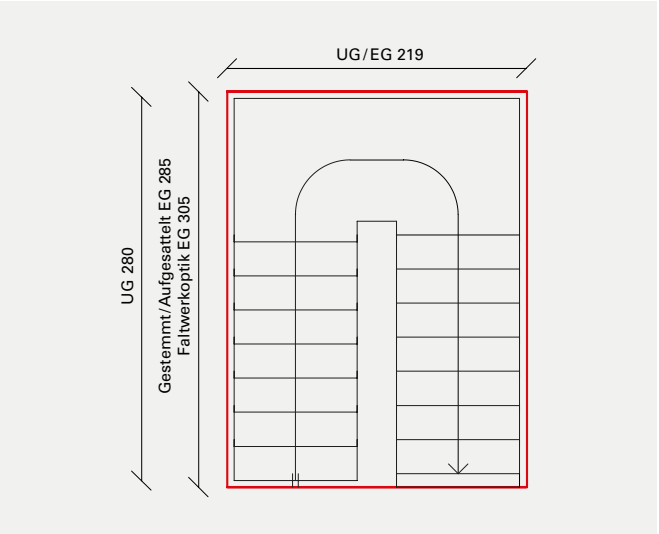
1 x 1/2 gewendelte Treppe, 2-läufige Podesttreppe
