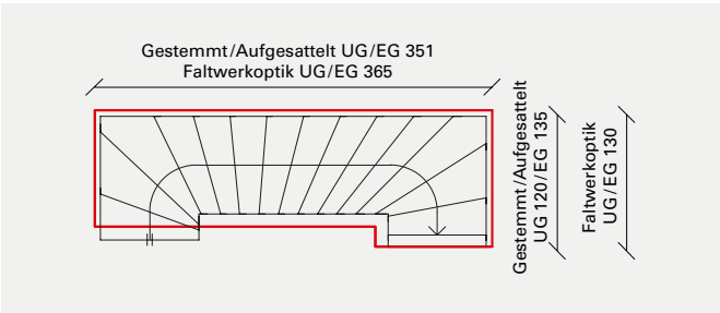
2 x 1/4 gewendelte Treppe
